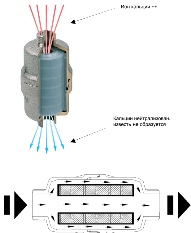
Схема прохода воды через магнитный нейтрализатор
